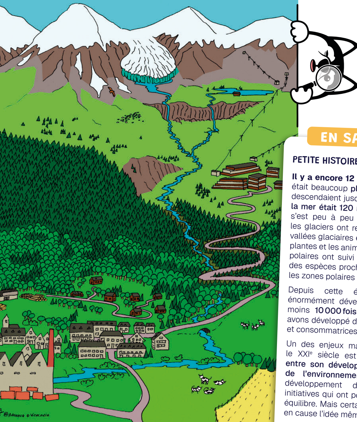
Schéma de l'écosystème alpin
