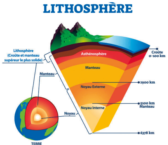
Schéma coupe de la Terre
